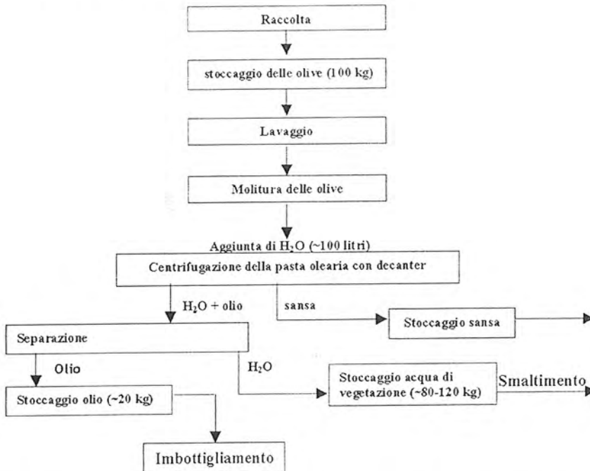
Schema 4 - Ciclo di estrazione continuo (per centrifugazione)
