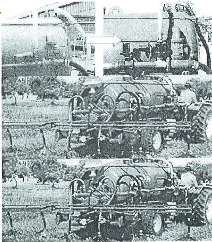
Foto 1 - Prototipo di carro botte per lo spargimento delle A.V.
