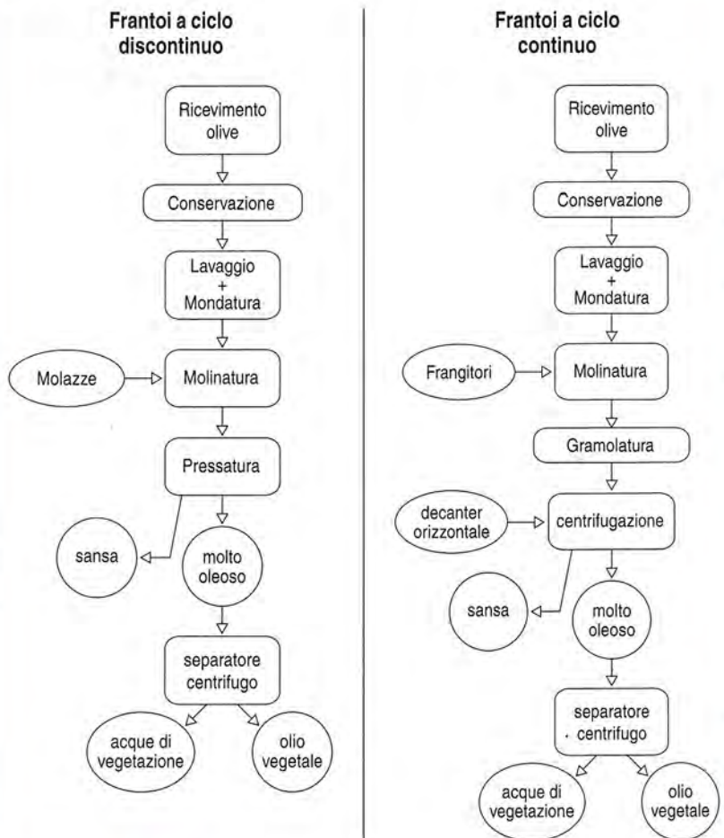
FIGURA 2 Rappresentazione schematica delle linee di estrazione olearia, a ciclo «discontinuo» (estrazione per pressione) oppure a ciclo «continuo» (estrazione per centrifugazione)
