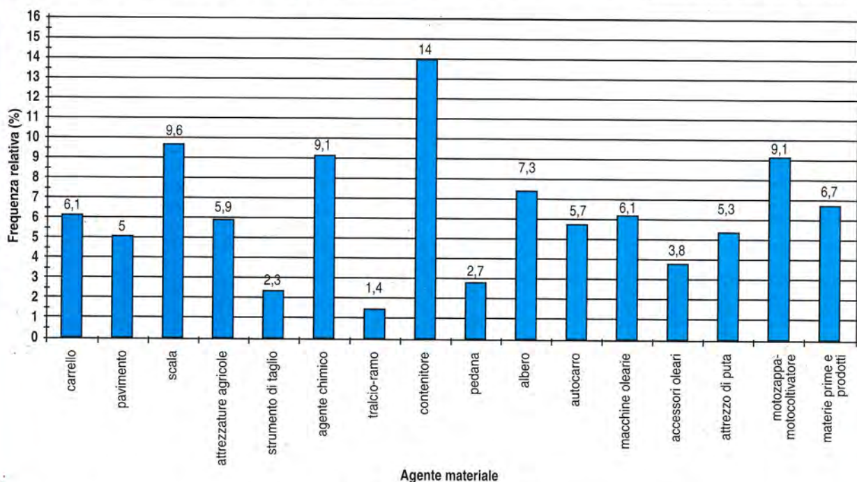
FIGURA 5 - Frequenza relativa della durata media degli infortuni suddivisi per agente materiale
